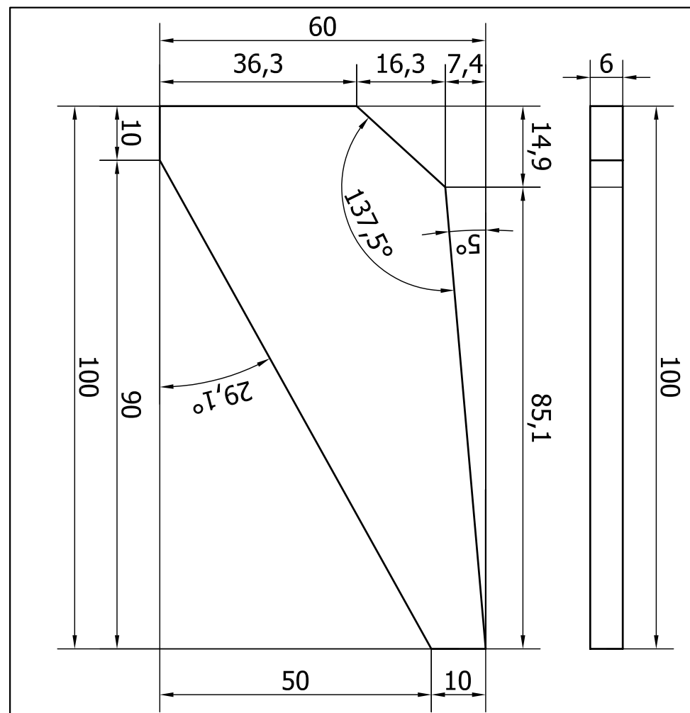
POS.19 SCALA ( 1:1 )
