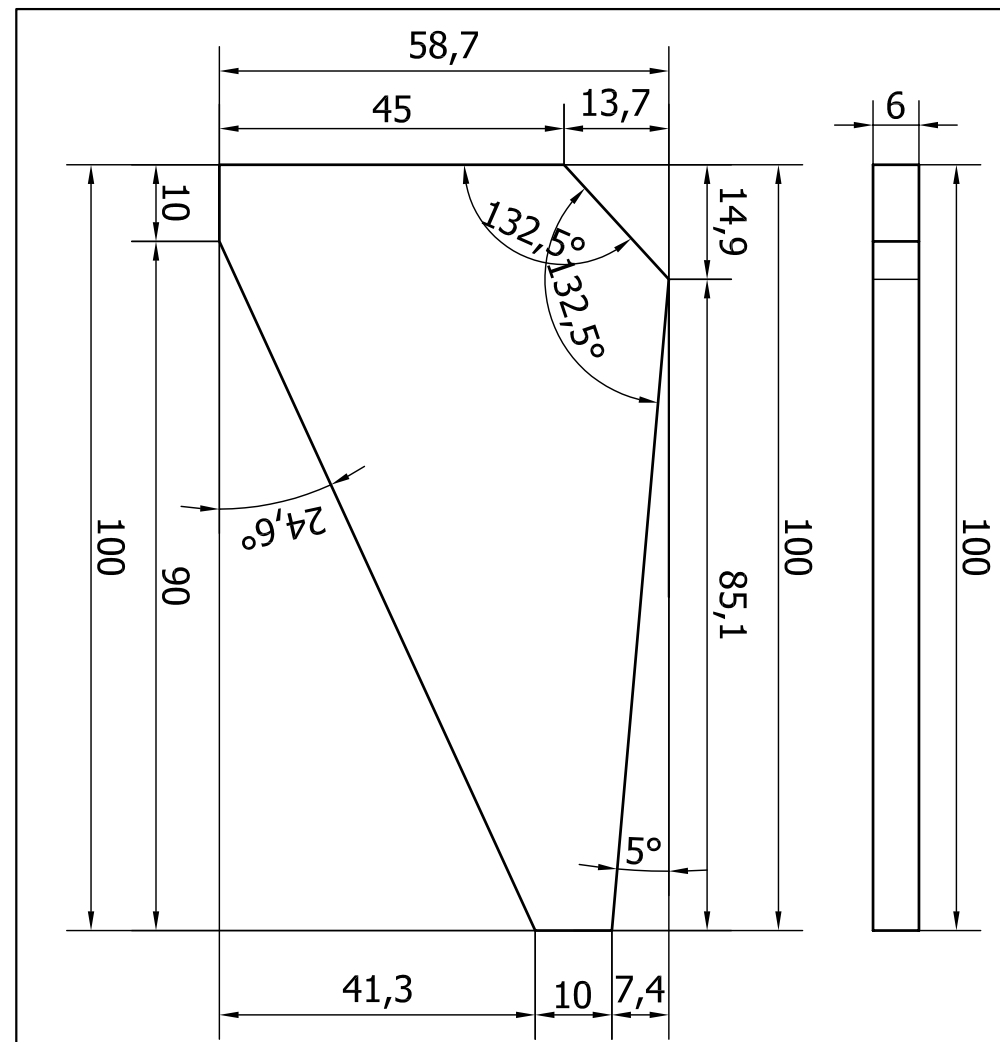
POS.20 SCALA ( 1:1 )
