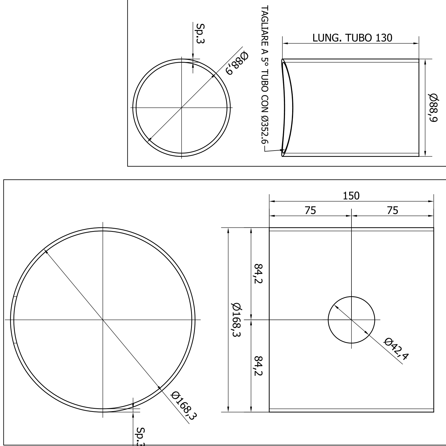
POS.5 SCALA ( 1:2 )
