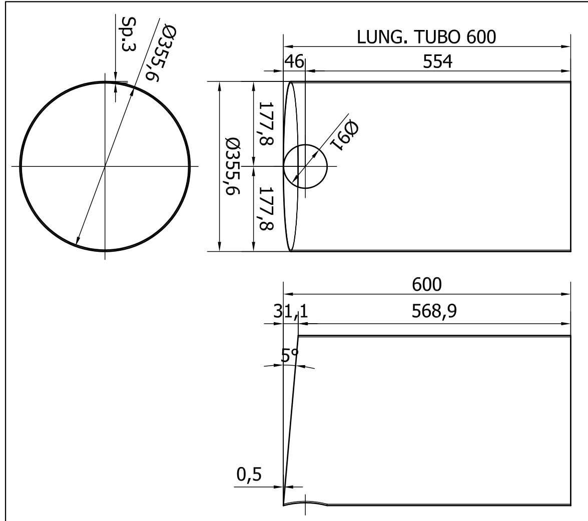
POS.14 SCALA ( 1 : 8 )
