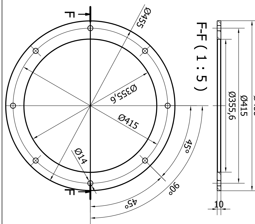
POS.16 SCALA ( 1 : 5 )
