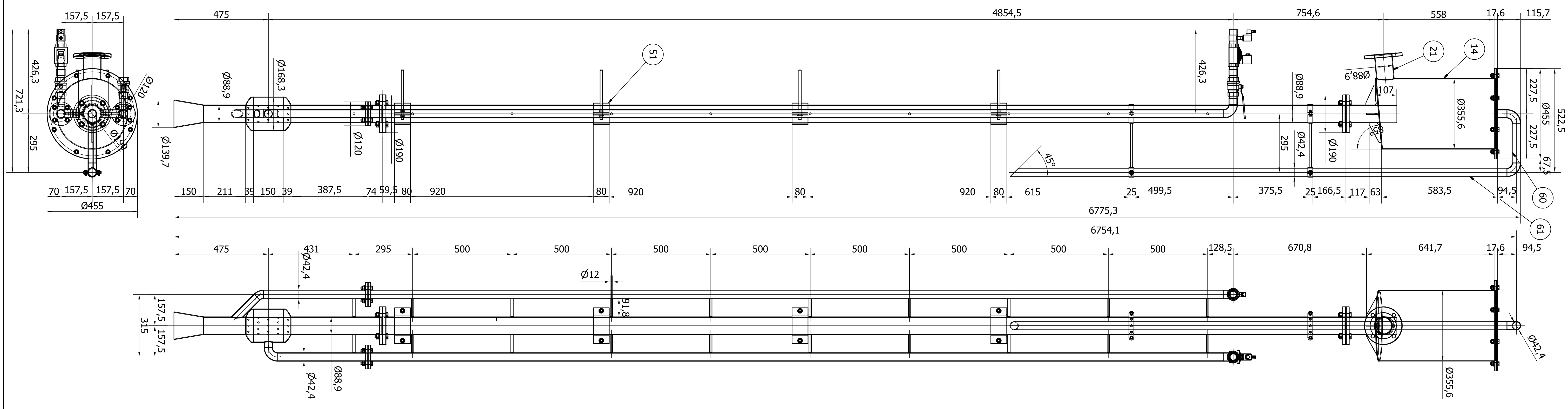
POS.19 SCALA ( 1:1 )
