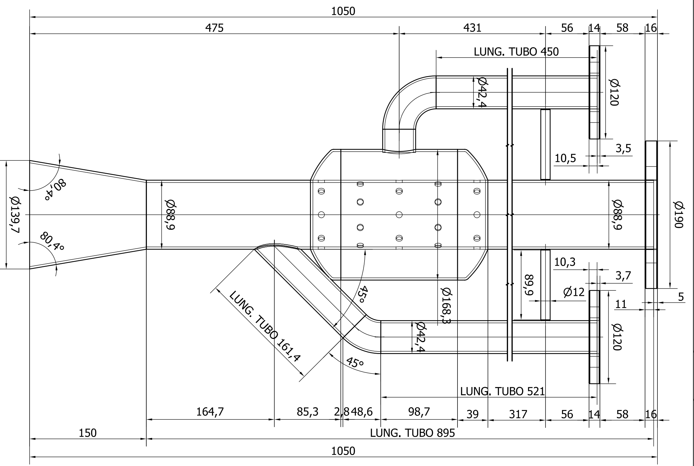
POS.9 SCALA ( 1:2 )
