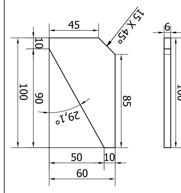
POS.18 SCALA ( 1:2 )
