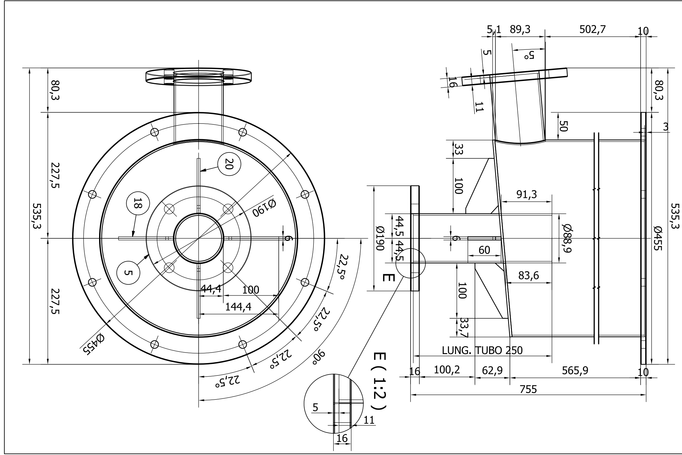
POS.21 SCALA ( 1:2 )
