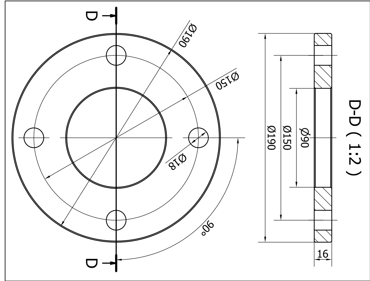
POS.5 SCALA ( 1:2 )
