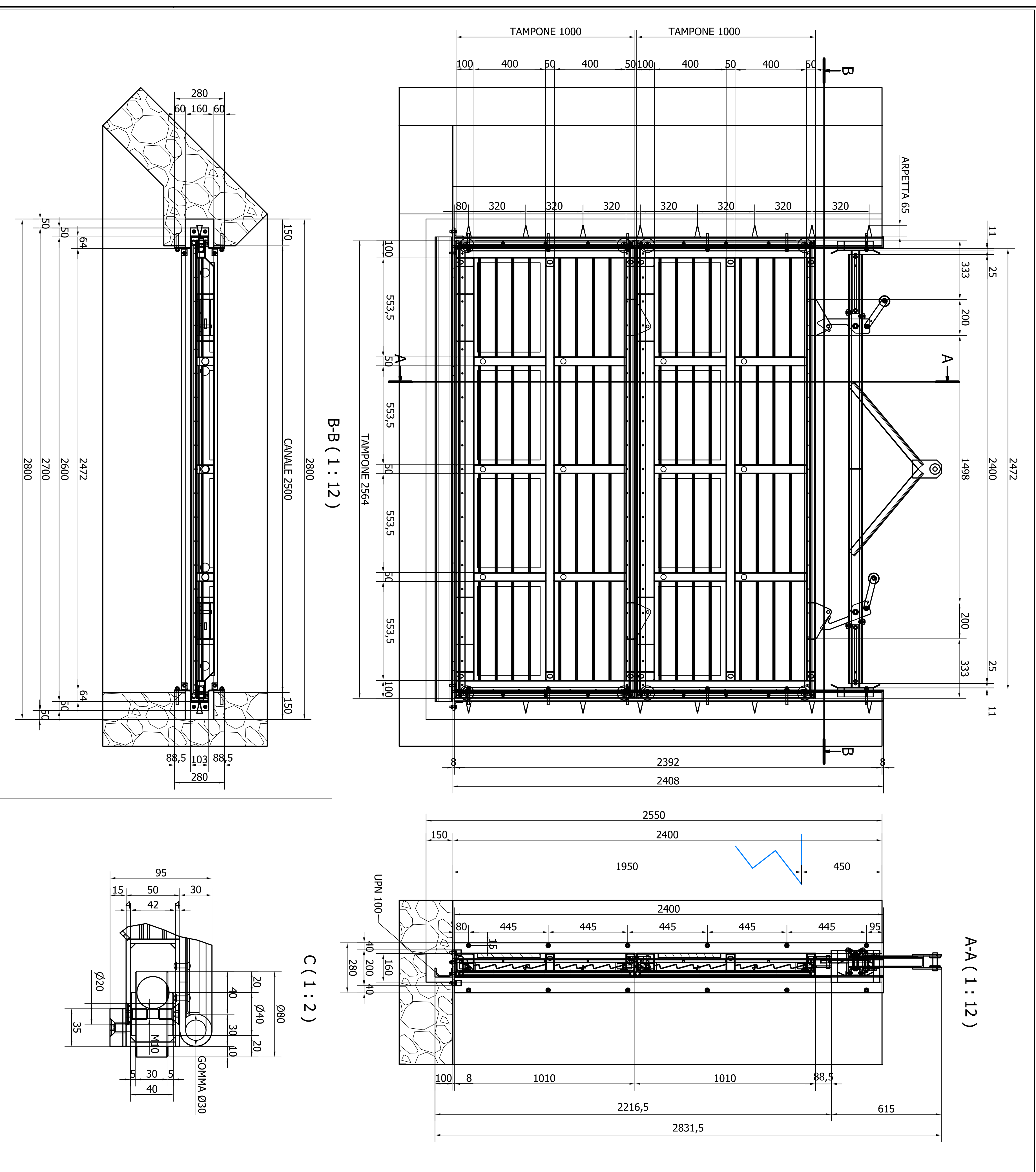
ASSIEME TAMPONE SCALA ( 1 : 8 )
