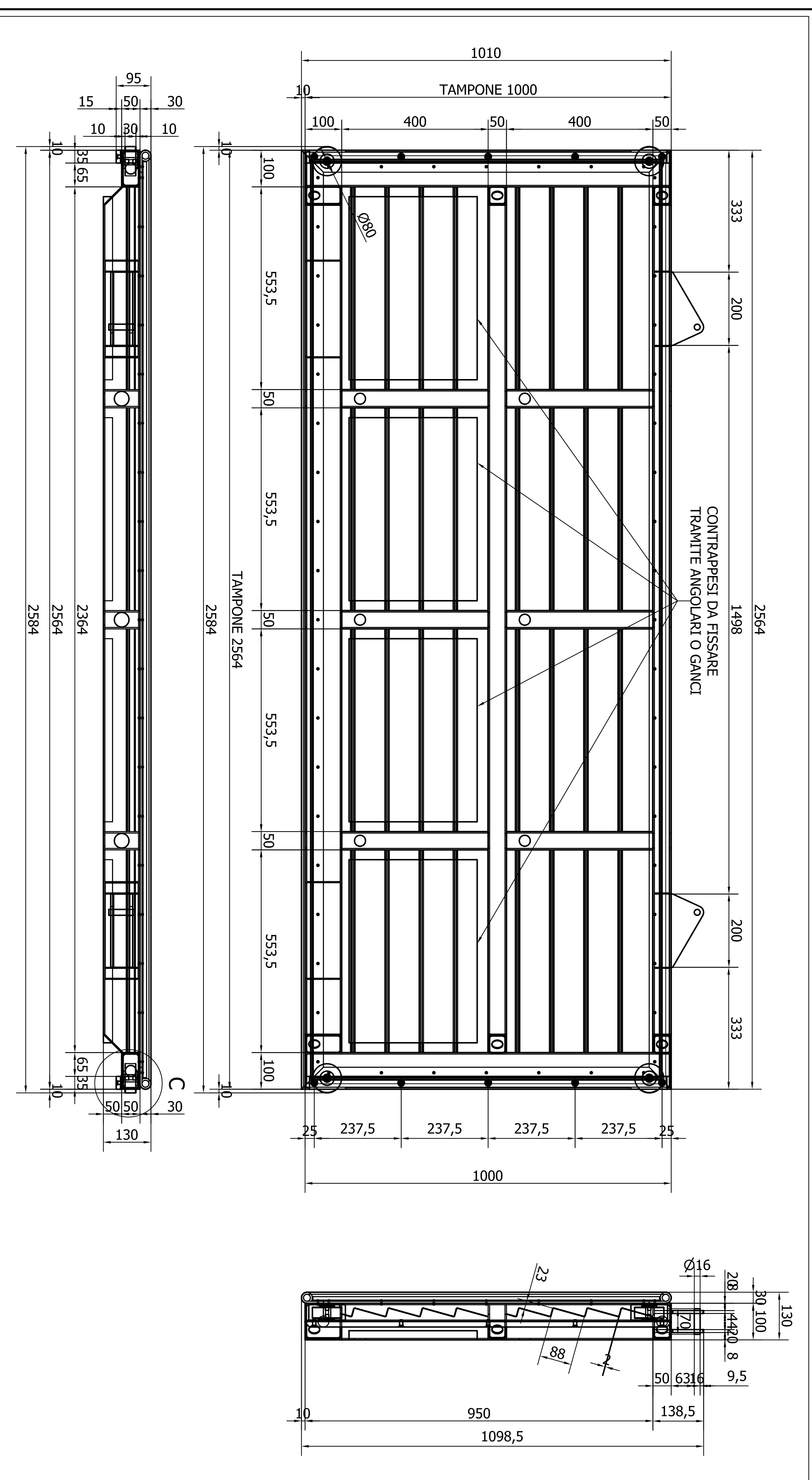
ASSIEME TAMPONE SCALA ( 1 : 8 )
