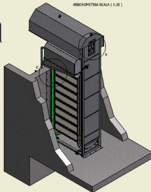
ASSONOMETRIA SCALA [ 1:20 ]
